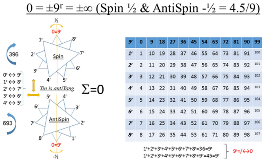
Fig.1. Spin & Antispin
